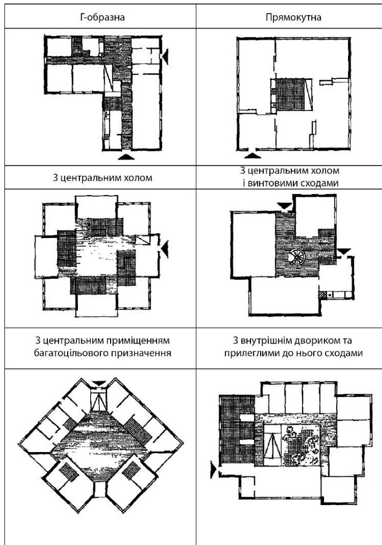
Рис. 1. Планувальні схеми блок-квартир дитячих будинків сімейного типу
