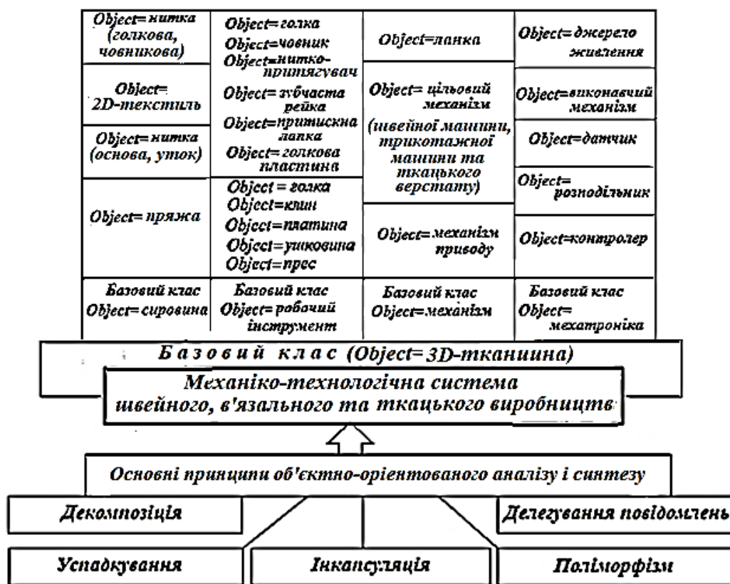
Рис. 1 – Схема узагальненої топології об'єктно-орієнтованого проектування механіко-технологічних систем 3D-тканин швейного, в'язального, ткацького та плетельного промислових виробництв
