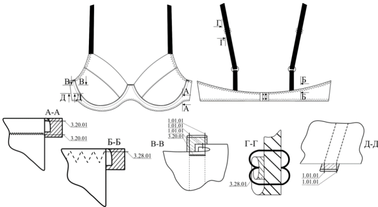
Рис. 1. Технічний рисунок бюстгальтера жіночого та його методи обробки тасьмою
