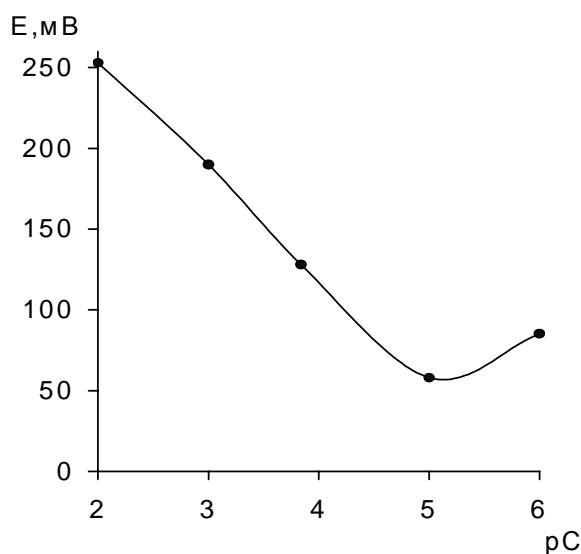
Рис. 7. Графічна залежність потенціалу іонселективного електроду від логарифма концентрації окситетрацикліну E=f(pC) (pH 7,0)
