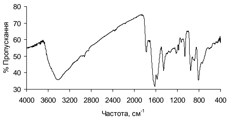
Рис. 6. ІЧ спектр поглинання (ІОТЦ) 3 РМо 12 О 40
