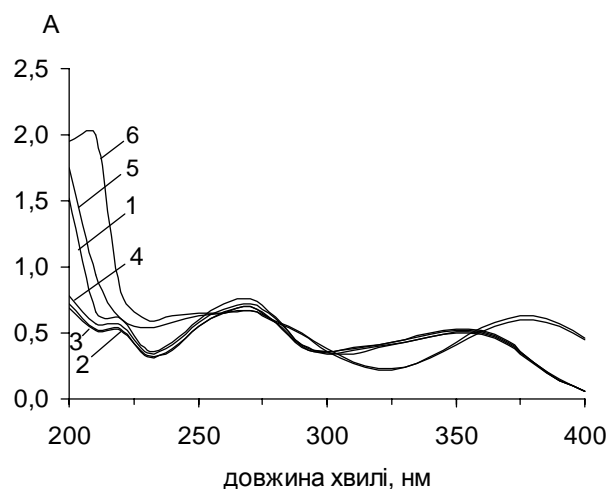
Рис. 2. Уф-спектри поглинання розчинів окситетрацикліну гідрохлориду при рН 1 (1); 4 (2); 5–6 (3); 8 (4); 10 (5); 12 (6).
