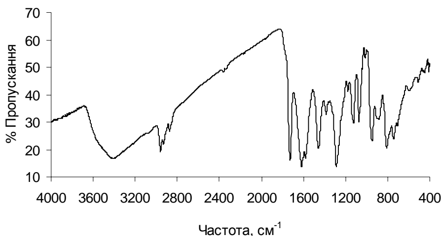
Рис. 5. ІЧ спектр поглинання (ОТЦ) 3 РМо 12 О 40
