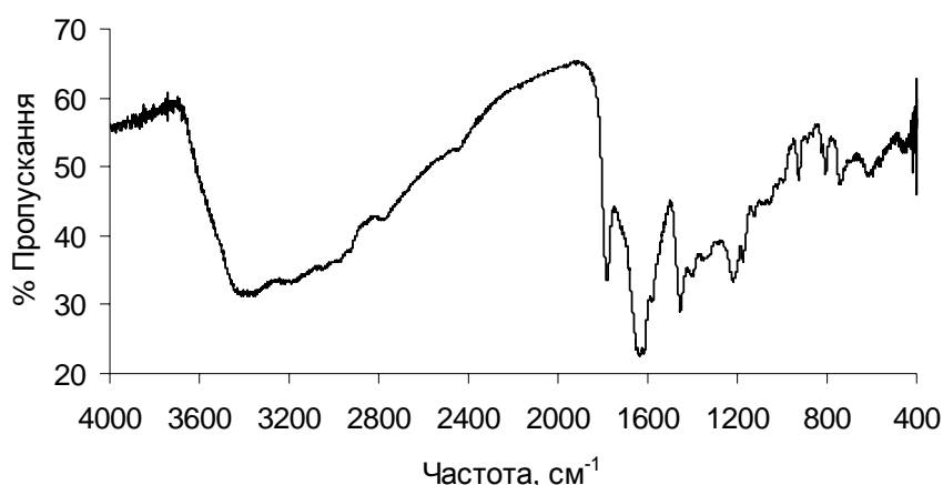
Рис. 4. ІЧ спектр поглинання ОТЦ гідрохлориду після термічної обробки
