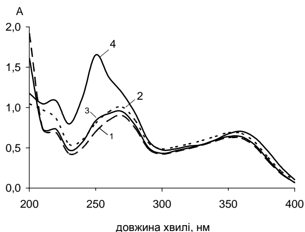
Рис. 1. Уф-спектри поглинання розчинів окситетрацикліну гідрохлориду після нагрівання до різних температур.
