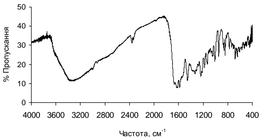
Рис. 3. ІЧ спектр поглинання ОТЦ гідрохлориду
